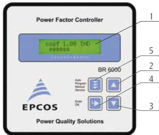
Рисунок 6. Передняя панель регулятора реактивной мощности
