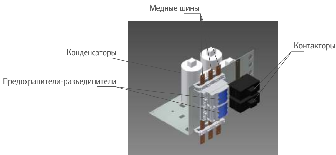
Рисунок 2. Внешний вид модулей для установок серии VARHET-AФ
