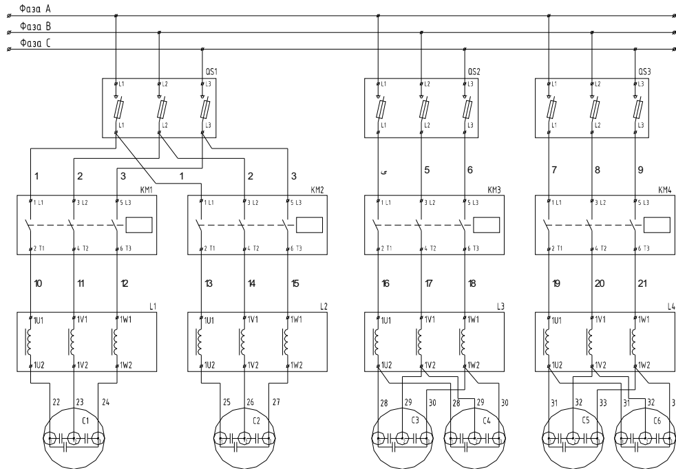
Схема электрическая принципиальная блока конденсаторного 2x25 + 2x50 кВар
