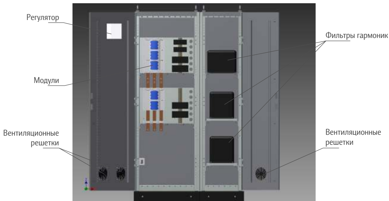
Рисунок 1. Внешний вид установок серии ВАРНЕТ-АФ
