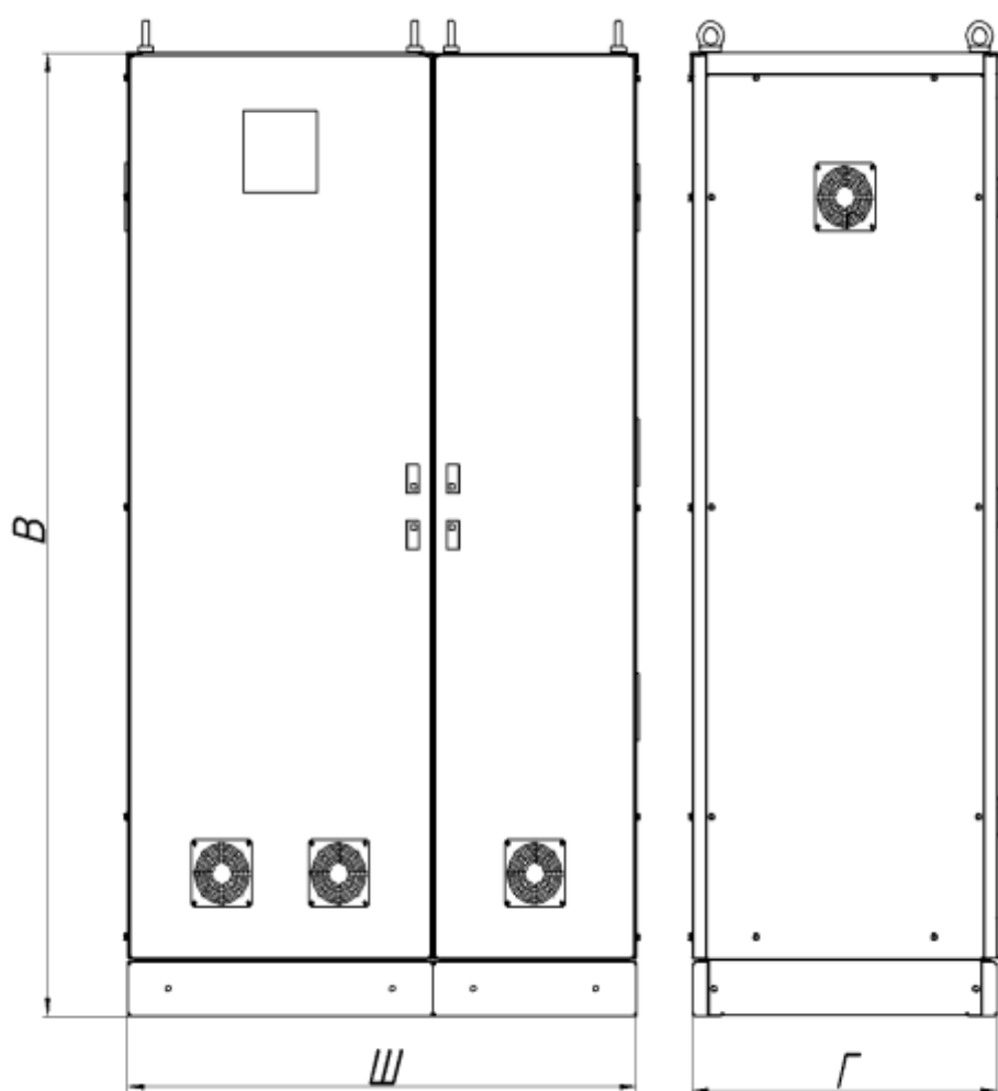
Рис.10 Габаритный чертеж установок ВАРНЕТ-АФ.
